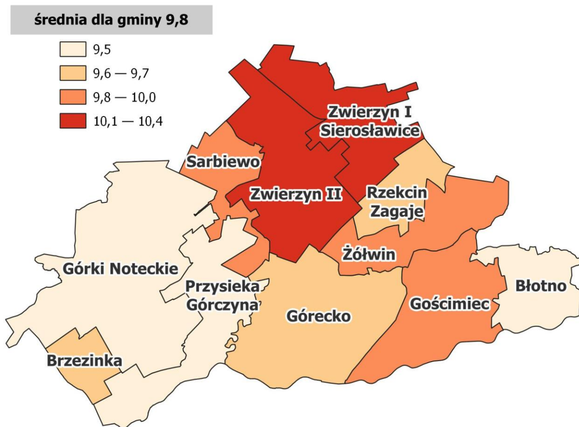
Rysunek 17. Średnie roczne stężenie PM2.5
