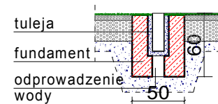
FUNDAMENT POD TULEJE DO ZESTAWU DO SIATKÓWKI skala 1:50
