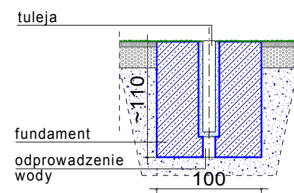
FUNDAMENT POD TULEJE DO ZESTAWU DO KOSZYKÓWKI skala 1:50
