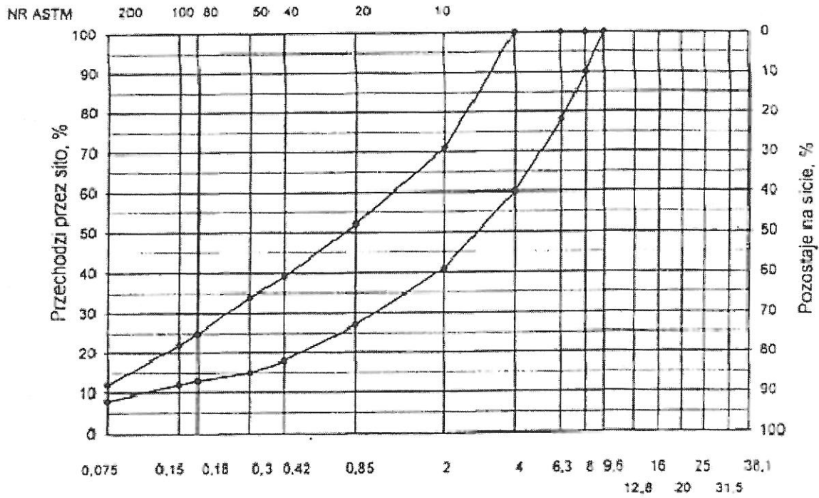
Rys. 3. Krzywe graniczne uziarnienia mieszanki mineralnej BA od 0 do 8mm, od 0 do 6,3 mm do warstwy ściernalnej nawierzchni drogi o obciążeniu ruchem nawierzchni drogi o obciążeniu ruchem KRI lub KR2
